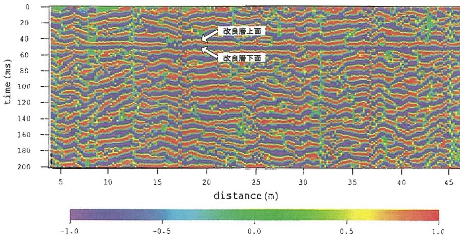
図-6 複素地震トレース解析の位相特性記録
