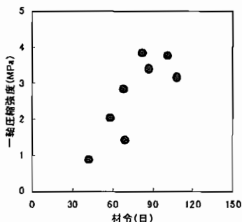
図-2 一軸圧縮強度と材令の関係
