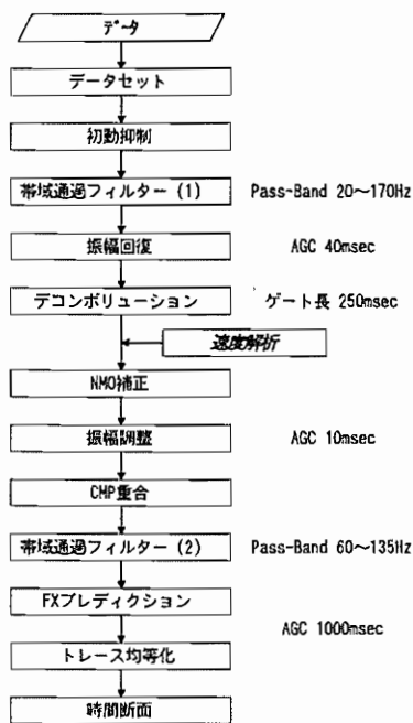
図-3 受振記録の処理の流れ
