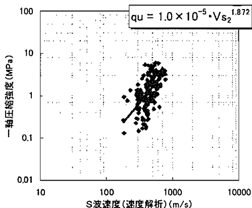
図-7 一軸圧縮強度とS波速度の関係
