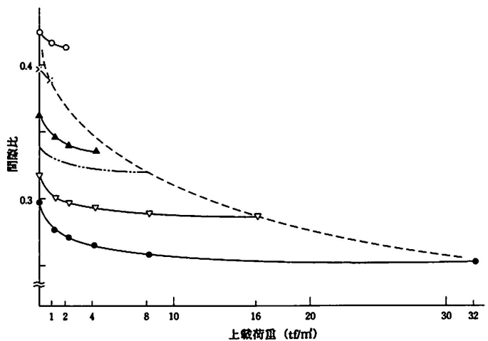
図5.2.11 蛇紋岩の膨張試験結果 20)
