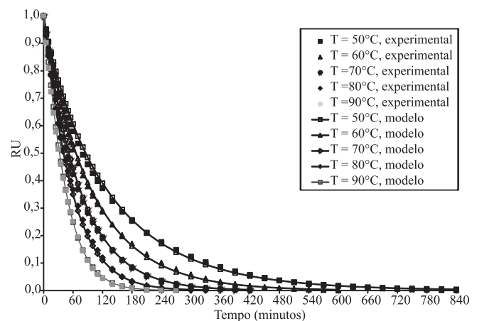
Figura 1. Curvas experimentais da secagem de camada delgada de bagaço de uva fermentado em função do tempo, previstas pelo modelo de Page modificado, a diferentes temperaturas. A razão de umidade (RU) foi calculada como RU = (U - U_e)/(U_o - U_e) , em que: U é a umidade em determinado tempo (em base seca); U_e é a umidade de equilíbrio (em base seca); e U_o é a umidade inicial (em base seca).
