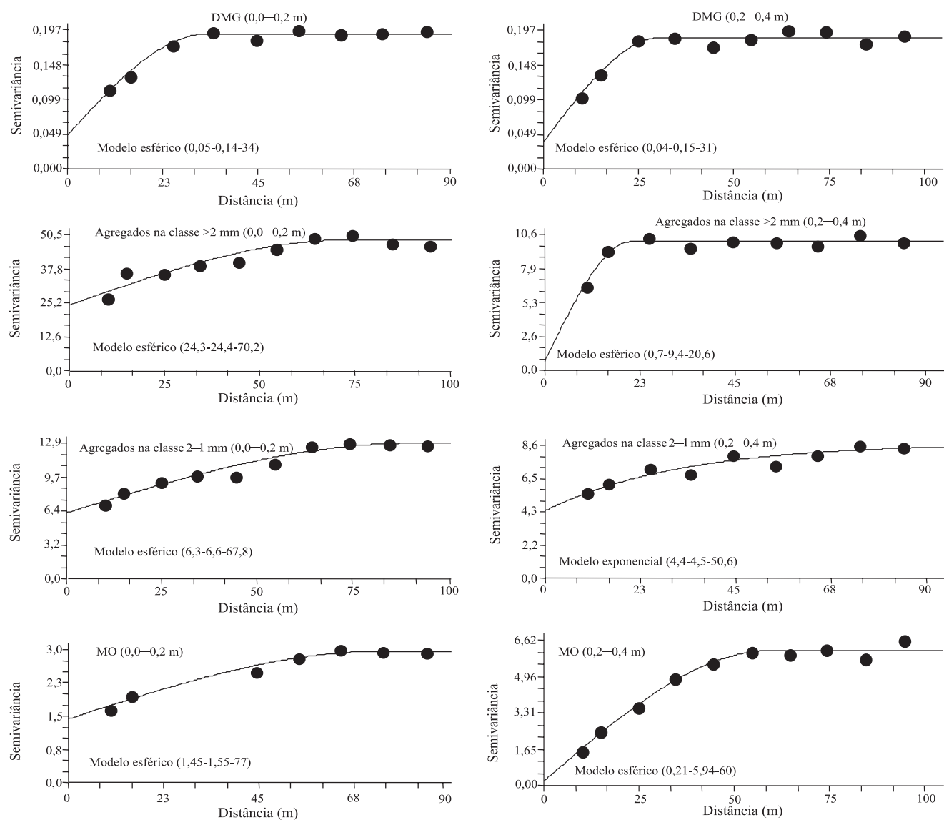
Figura 2. Semivariogramas das variáveis diâmetro médio geométrico (DMG, mm), agregados na classe >2 mm (%), agregados na classe 2–1 mm (%) e MO (g dm -3 ) nas profundidades de 0,0–0,2 m e 0,2–0,4 m, determinados pelos modelos ajustados esférico e exponencial (C 0 : efeito pepita; C = C 0 + C 1 : patamar; a: alcance).
