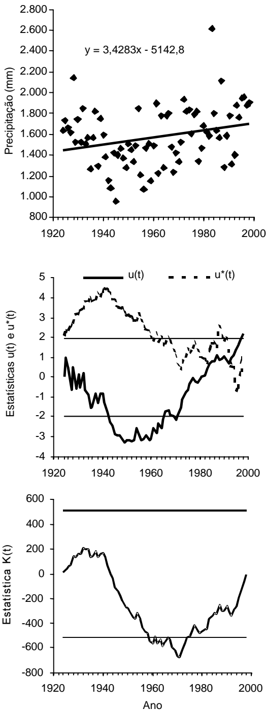
Figura 1. Precipitação total anual (regressão linear), estatísticas u(t) e u^*(t) do teste de Mann-Kendall e estatística K(t) do teste de Pettitt. As linhas horizontais representam o intervalo de confiança de 95%.
