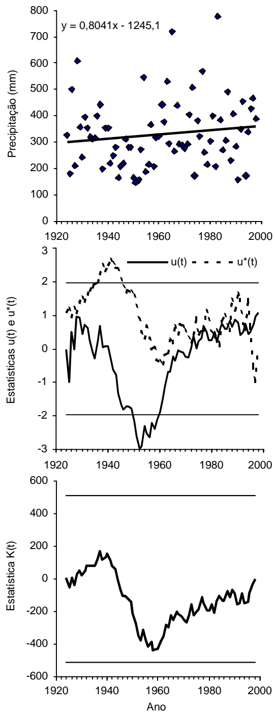
Figura 4. Precipitação total no terceiro trimestre (regressão linear), estatísticas u(t) e u^*(t) do teste de Mann-Kendall e estatística K(t) do teste de Pettitt. As linhas horizontais representam o intervalo de confiança de 95%.
