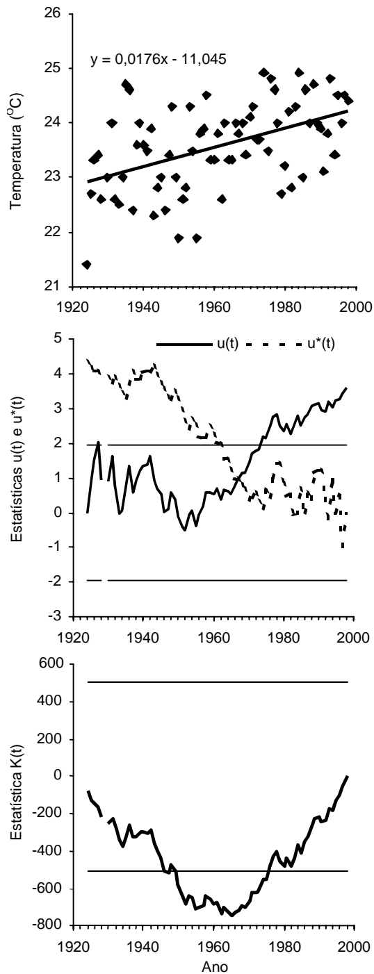
Figura 7. Temperatura média do mês de janeiro (regressão linear), estatísticas u(t) e u^*(t) do teste de Mann-Kendall e estatística K(t) do teste de Pettitt. As linhas horizontais representam o intervalo de confiança de 95%.
