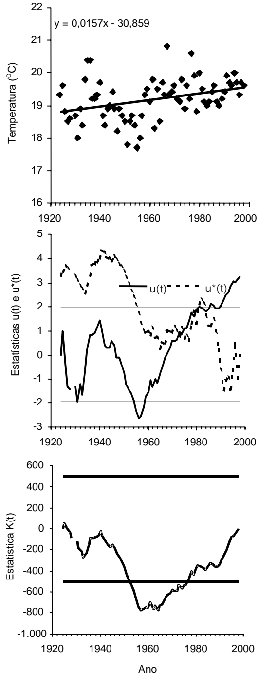
Figura 6. Temperatura média anual (regressão linear), estatísticas u(t) e u^*(t) do teste de Mann-Kendall e estatística K(t) do teste de Pettitt. As linhas horizontais representam o intervalo de confiança de 95%.
