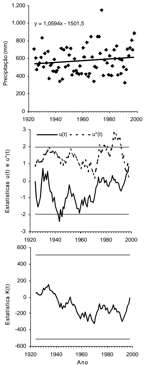
Figura 2. Precipitação total no primeiro trimestre (regressão linear), estatísticas u(t) e u^*(t) do teste de Mann-Kendall e estatística K(t) do teste de Pettitt. As linhas horizontais representam o intervalo de confiança de 95%.
