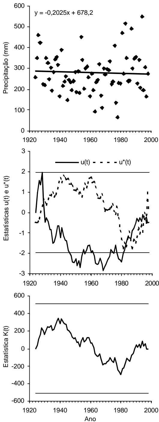
Figura 3. Precipitação total no segundo trimestre (regressão linear), estatísticas u(t) e u^*(t) do teste de Mann-Kendall e estatística K(t) do teste de Pettitt. As linhas horizontais representam o intervalo de confiança de 95%.
