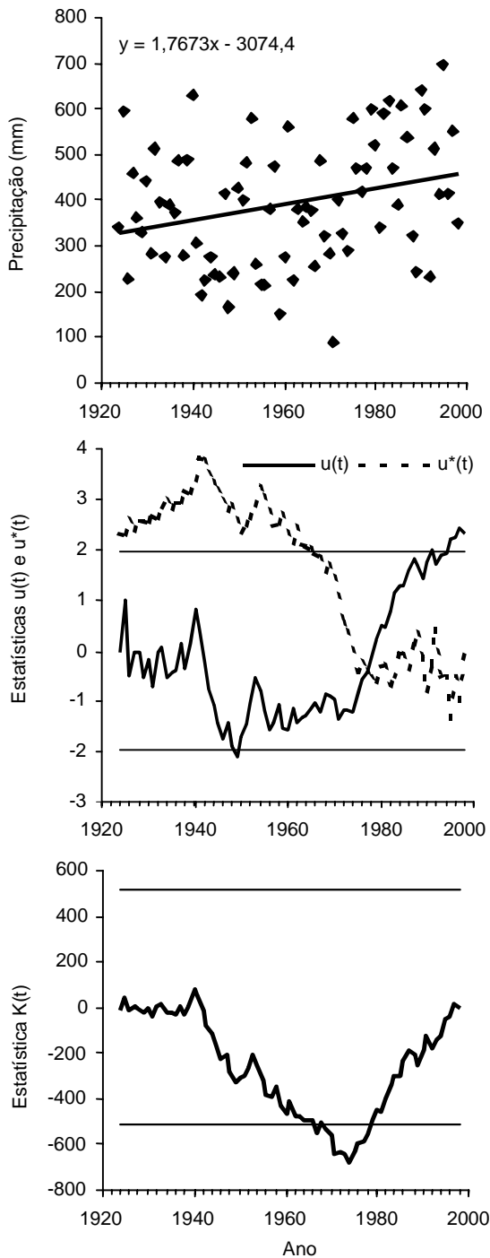
Figura 5. Precipitação total no quarto trimestre (regressão linear), estatísticas u(t) e u^*(t) do teste de Mann-Kendall e estatística K(t) do teste de Pettitt. As linhas horizontais representam o intervalo de confiança de 95%.
