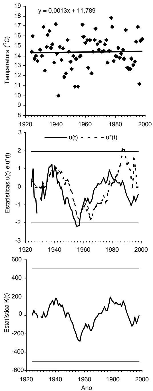
Figura 8. Temperatura média do mês de julho (regressão linear), estatísticas u(t) e u^*(t) do teste de Mann-Kendall e estatística K(t) do teste de Pettitt. As linhas horizontais representam o intervalo de confiança de 95%.
