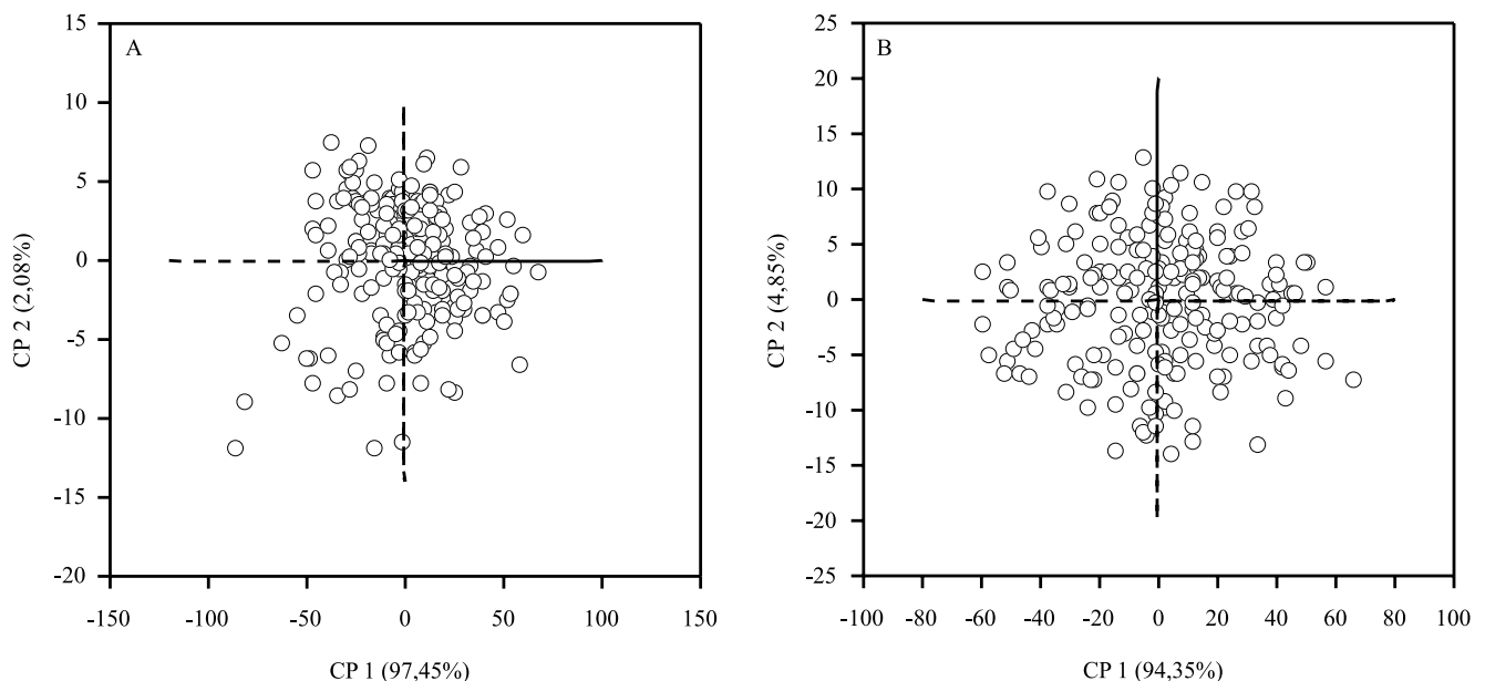
Figura 3. Resultados da ACP, com a distribuição dos espectros do conjunto de solos para as amostras de 2,0 mm (A) e 0,2 mm (B).
