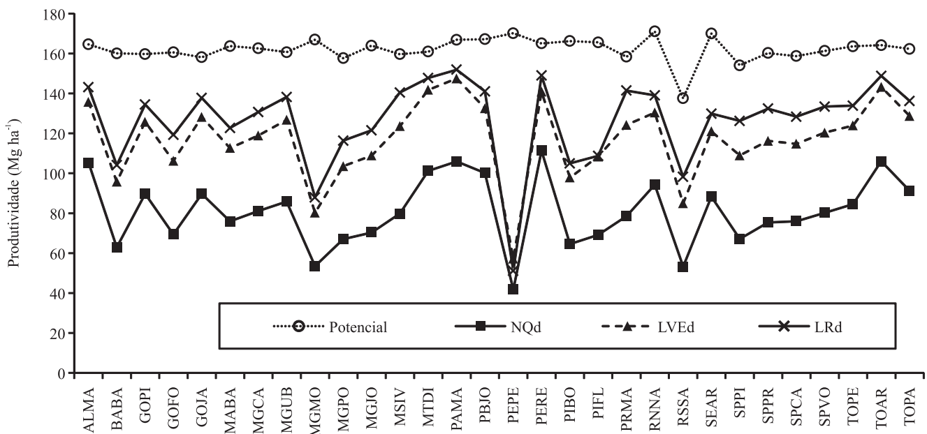
Figura 2. Produtividades potencial e atingível: médias para cada localidade, de acordo com o tipo de solo considerado (NQd, Neossolo Quartzarênico distrófico; LVEd, Latossolo Vermelho distroférico; LRd, Latossolo Vermelho distrófico). ALMA, Maceió, AL; BABA, Barreiras, BA; GOPI, Pirenópolis, GO; GOFO, Formosa, GO; GOJA, Jataí, GO; MABA, Balsas, MA; MGCA, Capinópolis, MG; MGUB, Uberaba, MG; MGMO, Mocambinho, MG; MGPO, Pompeu, MG; MGJO, João Pinheiro, MG; MSIV, Ivinhema, MS; MTDI, Diamantino, MT; PAMA, Marabá, PA; PBJO, João Pessoa, PB; PEPE, Petrolina, PE; PERE, Recife, PE; PIBO, Bom Jesus do Piauí, PI; PIFL, Floriano, PI; PRMA, Maringá, PR; RNNA, Natal, RN; RSSA, Santa Maria, RS; SEAR, Aracaju, SE; SPPI, Piracicaba, SP; SPPR, Presidente Prudente, SP; SPCA, Catanduva, SP; SPVO, Votuporanga, SP; TOPE, Peixe, TO; TOAR, Araguaína, TO; TOPA, Palmas, TO.
