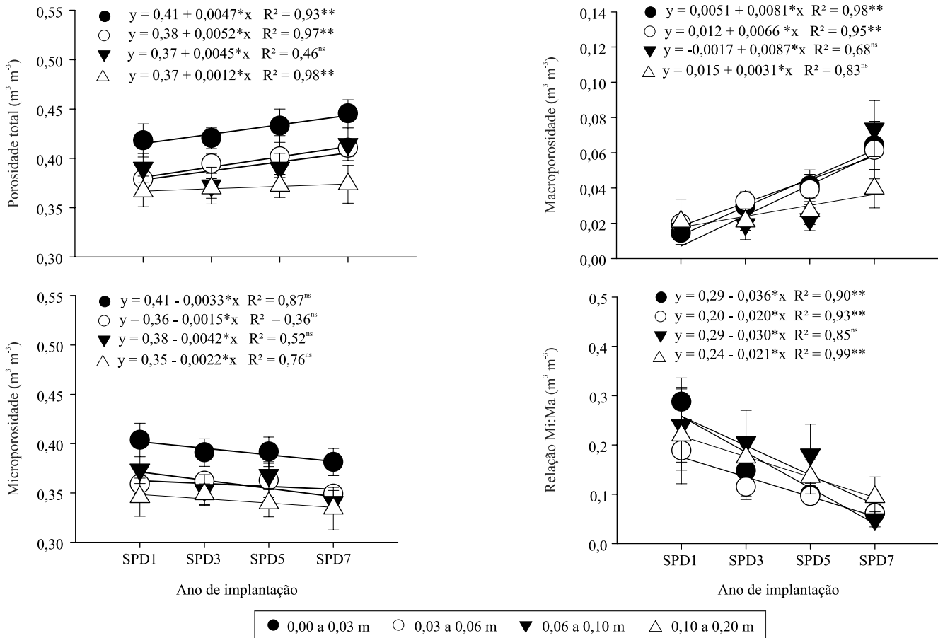
Figura 1. Porosidade total (Pt), macroporosidade (Ma), microporosidade (Mi) e relação Mi:Ma em um Planossolo Háplico sob diferentes tempos (T) de implantação do sistema plantio direto, nas diversas camadas do solo avaliadas. Barras verticais indicam os desvios em relação à média. ns Não significativo. * e **Significativo a 5 e 1% de probabilidade, respectivamente. SPD1, SPD3, SPD5 e SPD7 representam áreas com 1, 3, 5 e 7 anos de implantação do sistema plantio direto, respectivamente.
