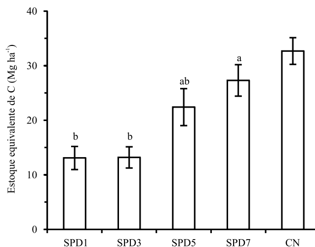
Figura 2. Estoque equivalente de carbono em Planossolo Háplico sob diferentes tempos de implantação do sistema plantio direto, e no campo não cultivado (CN). Médias seguidas de letras iguais não diferem pelo teste de Duncan a 5% de probabilidade. Barras verticais indicam os desvios em relação à média. SPD1, SPD3, SPD5 e SPD7 representam áreas com 1, 3, 5 e 7 anos de implantação do sistema plantio direto, respectivamente.
