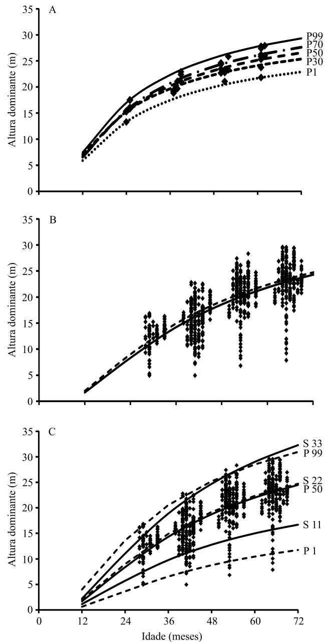
Figura 4. Curvas de índice de local, obtidas conforme as equações ajustadas pela regressão quantílica para diferentes percentis – P 1 , P 30 , P 50 , P 70 , P 99 – (A). Tendência de crescimento em altura dominante, a partir das equações ajustadas pelo método dos mínimos quadrados ordinários (linha contínua) e pela regressão quantílica (linha tracejada), para o banco de dados com 261 parcelas permanentes (B). Curvas de índice de local obtidas pelo método dos mínimos quadrados ordinários (linhas contínuas) e regressão quantílica (linhas tracejadas), para o banco de dados com 261 parcelas permanentes (C). Os pontos indicam as alturas dominantes observadas em cada parcela e em cada medição.
