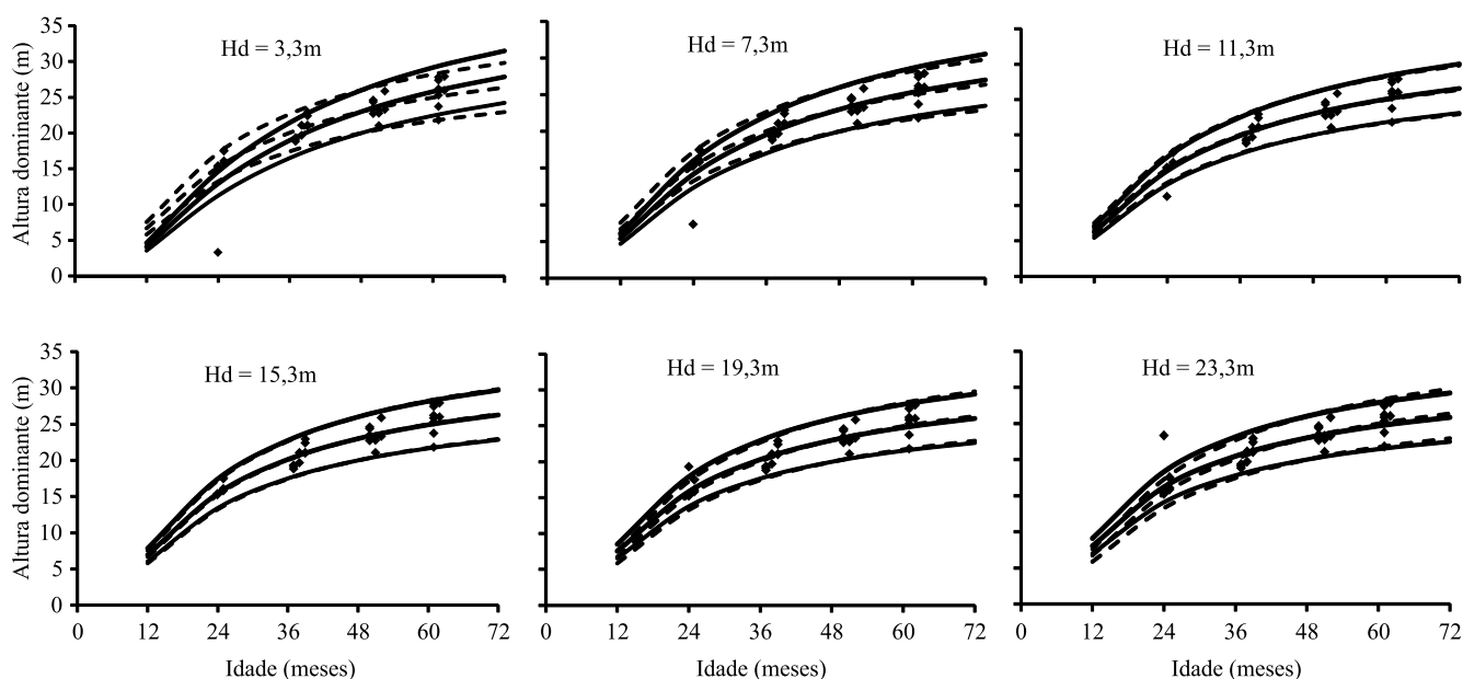
Figura 3. Curvas de índice de local, obtidas pelo método dos mínimos quadrados (linhas contínuas) e regressão quantílica (linhas tracejadas), com variação da altura dominante (Hd) em parcela com 24 meses. Os pontos indicam alturas dominantes observadas em cada parcela e em cada medição.
