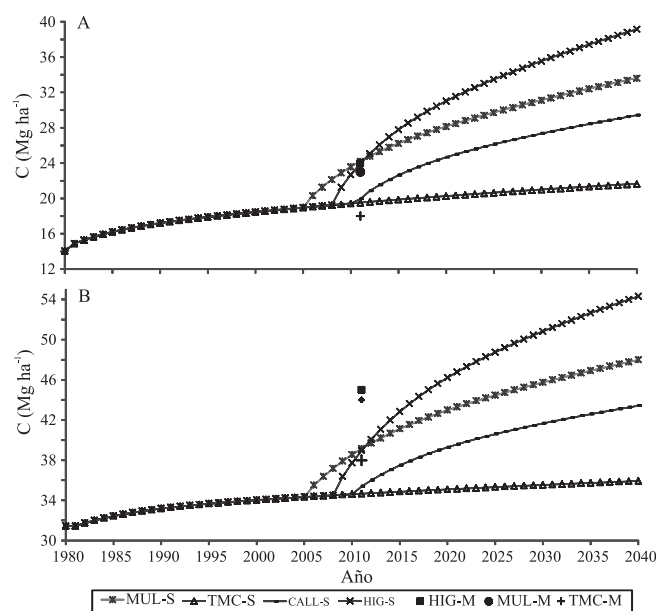
Figura 1. Carbono orgánico del suelo (COS) simulado con el RothC, en los sistemas: monocultivo de higuera multiestratos, callejones y tradicional maíz-calabaza, en un periodo de 60 años, en Santa María Roalo, Oaxaca, Mexico. A, simulación de COS para la profundidad 0–20 cm; B, simulación de COS para la profundidad 0–40 cm. TMC, sistema tradicional de la asociación maíz-calabaza; MUL, multiestratos; HIG, monocultivo de higuera; y CALL, callejones. –M, COS medido, y –S = COS simulado.
