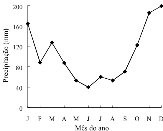
FIG. 1. Variação média da pluviosidade no município de Linhares, ES, no período de 1970-1995 (Fonte: Sexto distrito de meteorologia, EMCAPA/Linhares, ES).
