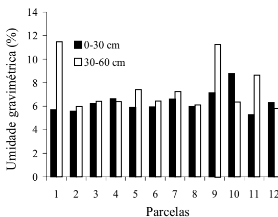
FIG. 2. Umidade do solo durante os testes de infiltração, no ano de 1994.
