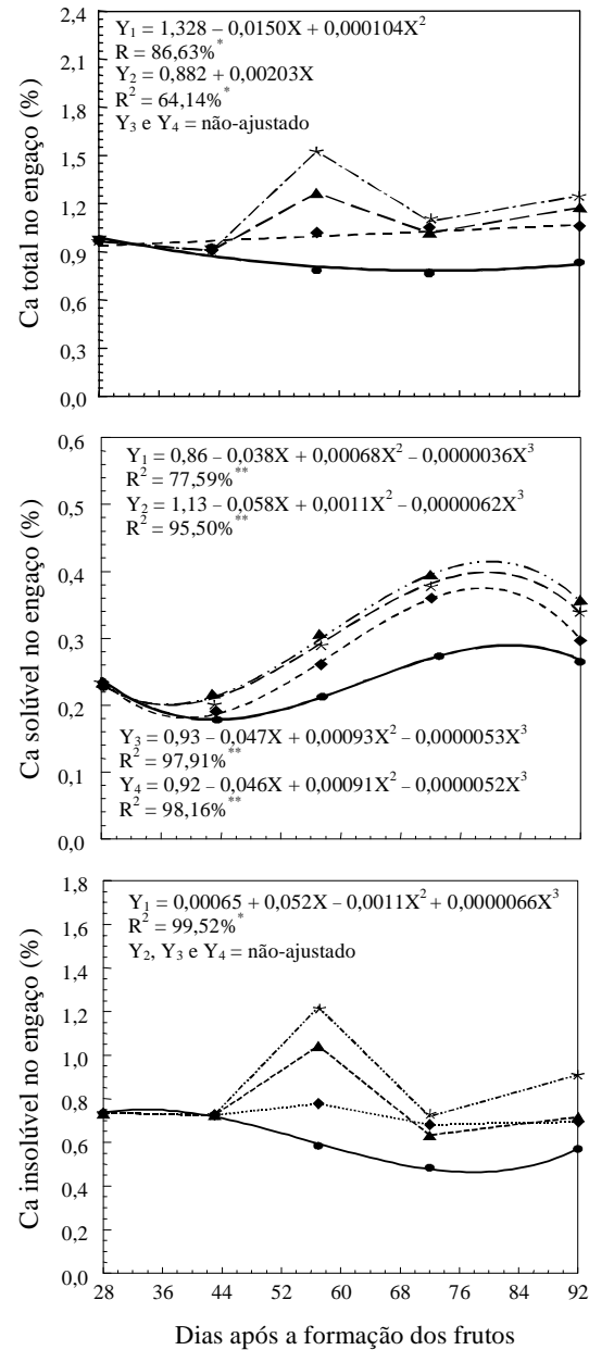
Figura 3. Teores de Ca total, Ca solúvel e Ca insolúvel no engaço de uva ‘Itália’ durante a fase de desenvolvimento e amadurecimento, em razão do tratamento aos 57 dias após a formação dos frutos, com solução a 0,0 ( y_1 ,●), 0,5 ( y_2 ,♦), 1,0 ( y_3 ,▲) e 1,5% ( y_4 ,*) de Ca.
