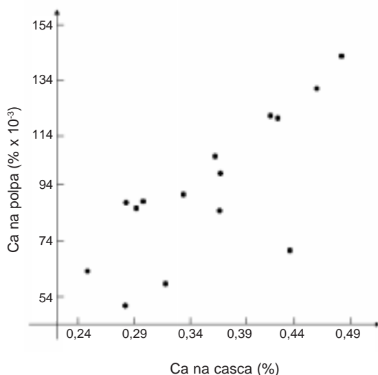
FIG. 1. Correlação entre o Ca na casca e Ca na polpa ( r^2 = 76,13\% ).
