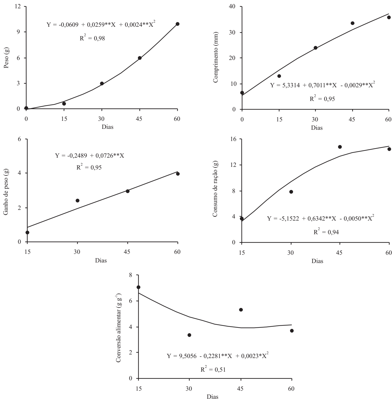
Figura 1. Peso, comprimento, ganho de peso, consumo de ração e conversão alimentar de girinos de rã-touro, alimentados com ração comercial com 32% de proteína bruta, durante 60 dias. * e **Significativo a 5 e 1% de probabilidade, respectivamente.
