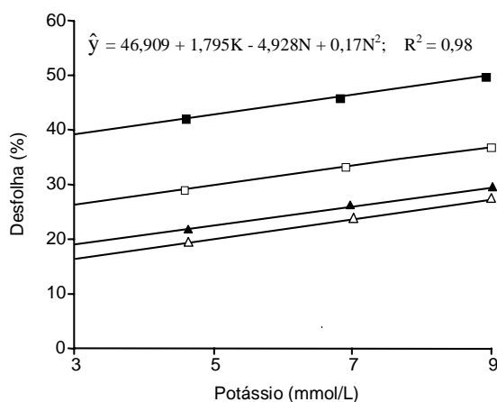
Figura 3. Porcentagem de desfolha causada por Cercospora coffeicola , em razão de doses de K em cada dose de N (3■, 7□, 11▲ e 15△ mmol/L), em solução nutritiva.
