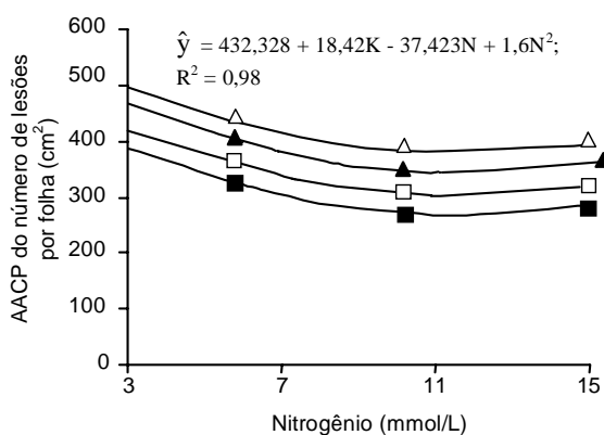
Figura 2. Área abaixo da curva de progresso (AACP) do número de lesões de Cercospora coffeicola por folha de café, em razão de doses de N em cada dose de K (3■, 5□, 7▲ e 9△ mmol/L), em solução nutritiva.
