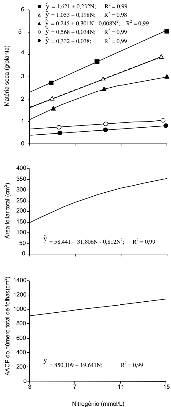
Figura 1. Produção de matéria seca total (■), da parte aérea (△), da folha (▲), da raiz (○) e do caule (●), área foliar total e área abaixo da curva de progresso (AACP) do número total de folhas de mudas de cafeeiro, em razão de doses de N, em solução nutritiva.
