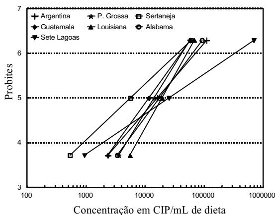
FIG. 1. Regressão entre o logaritmo da concentração de isolados geográficos de vírus de poliedrose nuclear e a probabilidade de mortalidade (Probites) de larvas de segundo instar de Spodoptera frugiperda .
