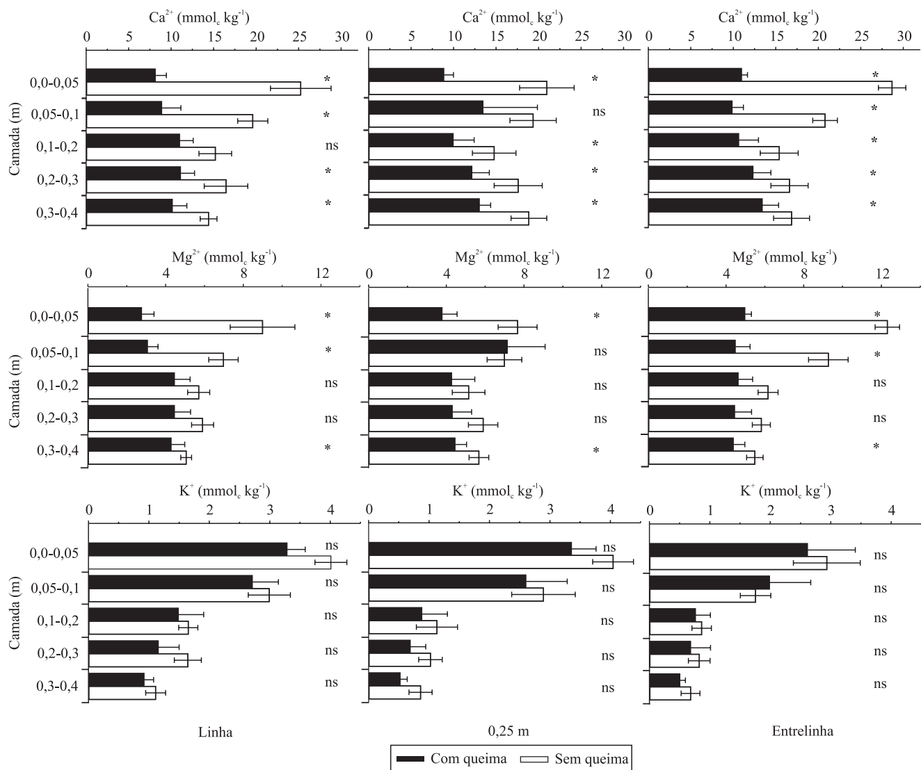
Figura 2. Teores de Ca 2+ , Mg 2+ e K + em Latossolo Vermelho distrófico sob colheita de cana-de-açúcar com e sem queima. ns Não significativo. *Diferenças significativas entre os sistemas com e sem queima pelo teste de Tukey, a 5% de probabilidade. As barras representam o erro-padrão da média.
