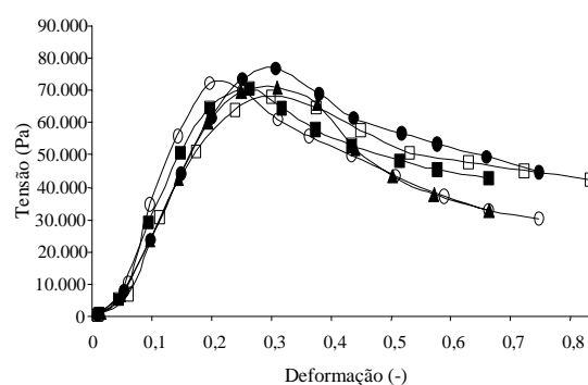
Figura 1. Curva de tensão ( T ) vs. deformação ( \epsilon H ) na ruptura de melão sem tratamento (fruta fresca) em cinco amostras (1: ●; 2: ○; 3: □; 4: ▲; 5: ■) provenientes de uma mesma fruta.
