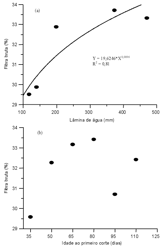
FIG. 4. Fibra bruta do capim-buffel (%) como resposta às lâminas totais de água(a) e à idade ao primeiro corte (b).
