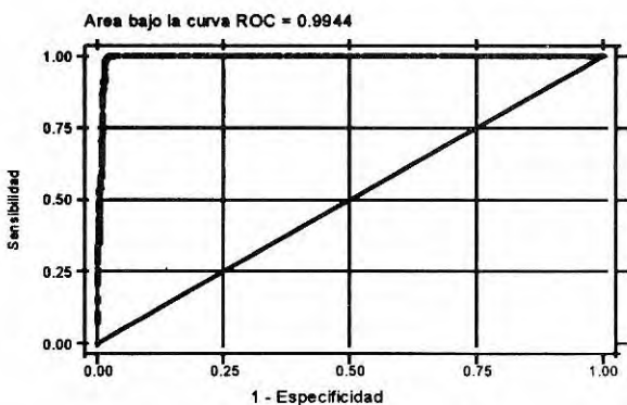
Figura 1. Area bajo la curva del receptor operador (ROC) de la prueba de ELISA
