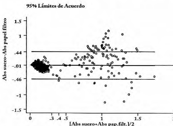
Figura 2. Límites de acuerdo del 95% utilizando el método de Bland y Altman entre las absorbancias del ELISA en suero y papel de filtro para la detección de anticuerpos contra Trypanosoma cruzi
