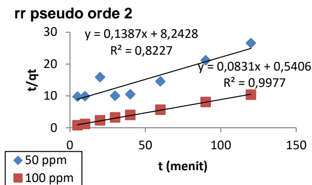
Gambar 4. Kurva kinetika adsorpsi pseudo orde-2 dari Reactive Red
