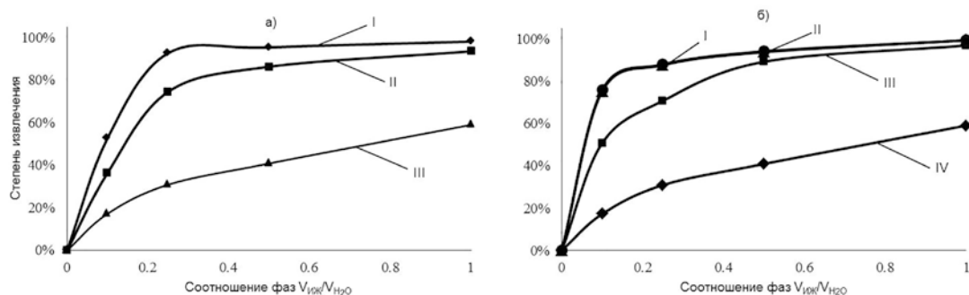
Рис. 2. (а) Зависимость степеней извлечения кортизола (F) в ионные жидкости от соотношения фаз ИЖ : водный раствор. I – C_8MlmBF_4 , II – C_6MlmBF_4 , III – C_6MlmNTf_2 ; (б) Зависимость степеней извлечения стероидных гормонов от соотношения C_8MlmBF_4 : водная фаза. I – 11-дезоксикортизол (S), II – кортикостерон (B), III – кортизон (E), IV – кортизол (F)
