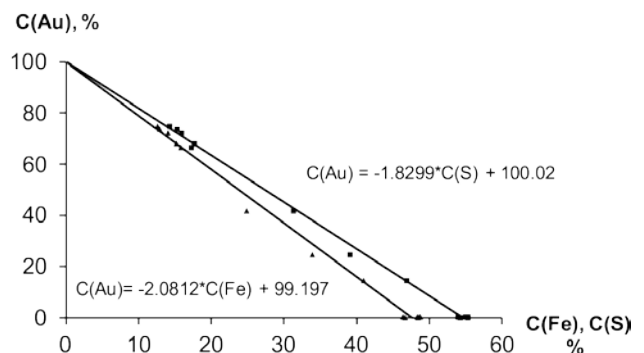
Рис. 6. Тренды содержаний золота в сравнении с содержаниями железа и серы, полученных при измерении состава торцевой части слоя золота, нанесенного на пирит. Коэффициент корреляции для обоих трендов составляет 0.99
