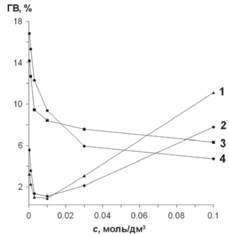
Рис. 5. Доля гумусовых веществ в элюате (ГВ, %) в зависимости от концентрации соли в природной воде: CuSO_4 (1), NiSO_4 (2), K_2SO_4 (3), Na_2SO_4 (4); m(Al_2O_3) = 2 г, V(\text{элюата}) = 20 см 3 .
