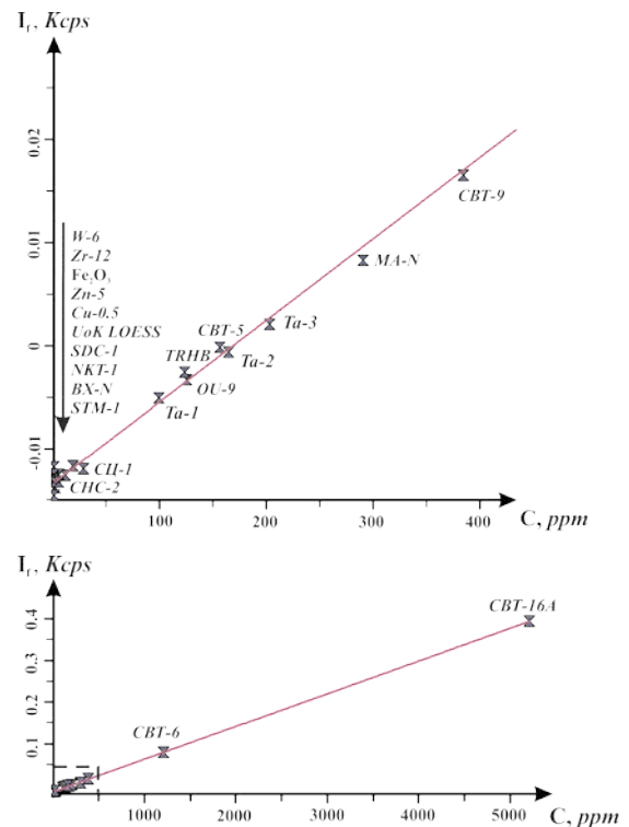
Рис. 3. Градуировочный график для Ta в диапазоне содержаний: а – от 2.6 до 400 ppm, б – от 400 до 5200 ppm Fig. 3. Calibration plots for the range of Ta contents: а – from 2.6 to 400 ppm, б – from 400 ppm to 5200 ppm
