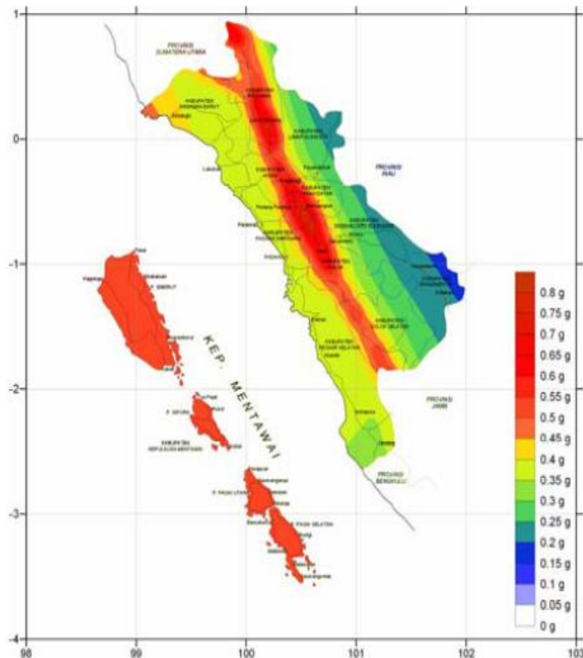
Gambar 2. Peta Zonasi Sumatera Barat, PBA untuk periode ulang 475 tahun(Sengara dkk, 2009)
