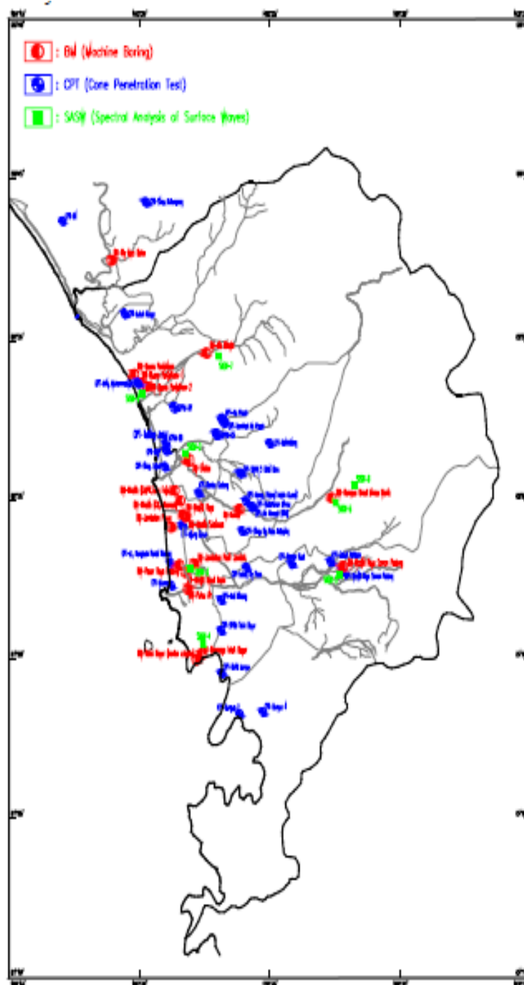
Gambar 3. Lokasi penyelidikan tanah yang dilakukan di Kota Padang (Sengara dkk, 2009)
