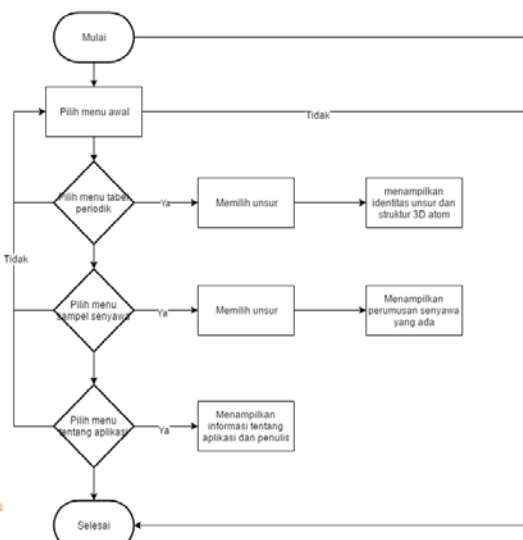
Gambar 5. Flowchart Tabel Periodik dan Perumusan Senyawa
