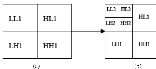
Gambar 2. Dekomposisi wavelet (a) level 1 dan (b) level 2
