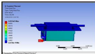
Fig.4.4. Heat flux.
