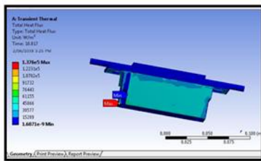
Fig.4.2. Heat flux
