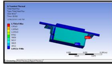
Fig.4.6. Heat flux
