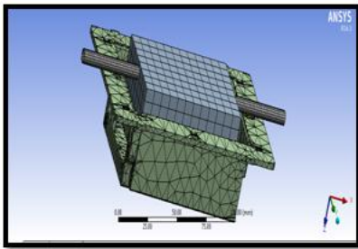
Fig.4.1. Meshed model.
