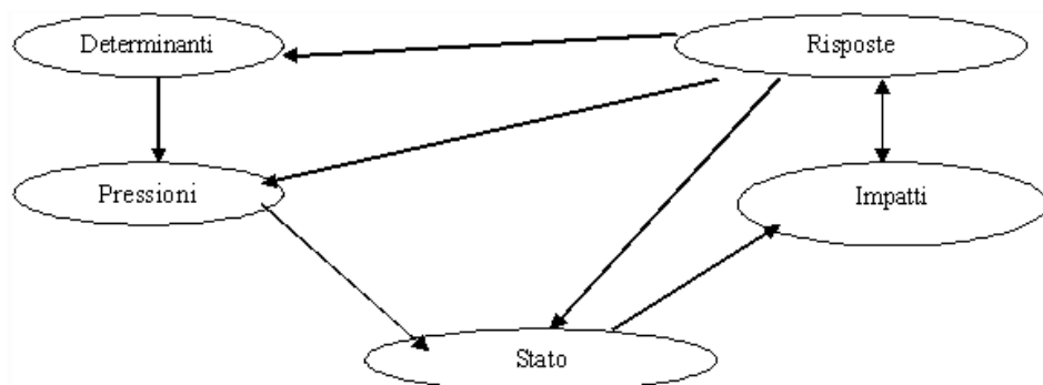
Figura 2. Modello DPSIR.
