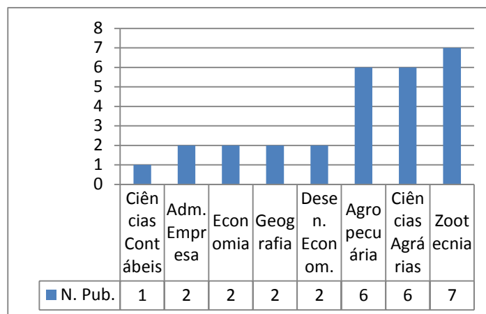
Figura 3 – Número de publicações por área de interesse
