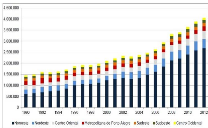
Figura 4 – Evolução da produção leiteira em regiões do RS
