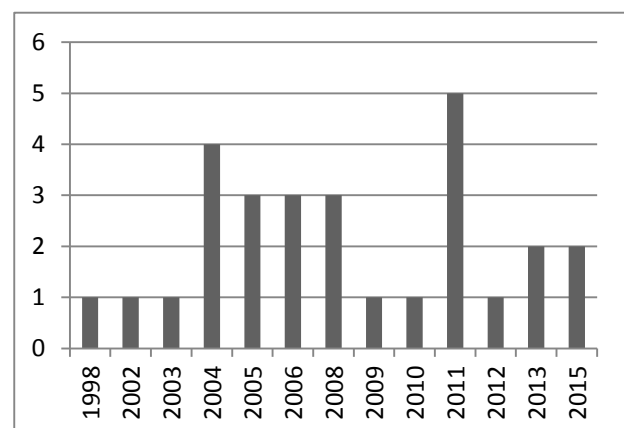
Figura 1 – Número de publicações por ano
