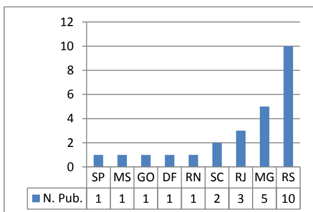
Figura 2 – Número de publicações por Estado do Brasil
