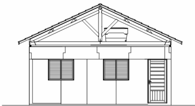
Figura 5 – Corte transversal do projeto desenvolvido
