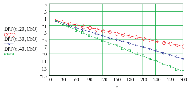
Gráfico N°9: Modelo para Diferencia de Peso de la Fruta Porcentual (DPF %) Tiempo (min) Para la mayor concentración de CSO=65°Brix, se grafica para tres temperaturas 20, 30 y 40°C.
