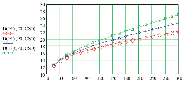
Gráfico N°8: Modelo de Diferencia de Concentración de la Fruta (DCF °Brix) vs. Tiempo (min). Para la mayor concentración de CSO=65°Brix, se grafica para tres temperaturas 20, 30 y 40°C.
