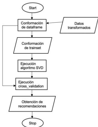
Figura 4. Modelo de recomendación.
