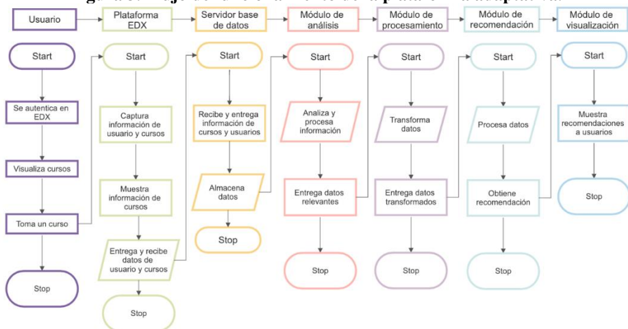
Figura 3. Flujo de funcionamiento de la plataforma adaptativa.
