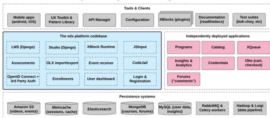
Figura 1. Arquitectura de Open EDX.
