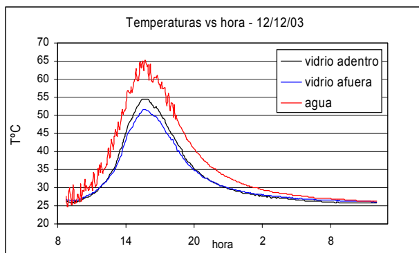
Figura 5. Temperatura del agua y del vidrio para el 12/12/03.
