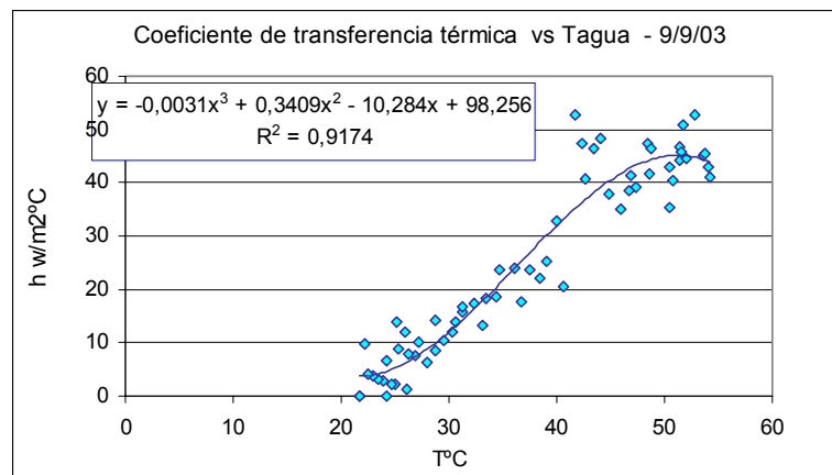
Figura 2. Coeficiente de transferencia térmica h en función de la temperatura del agua y ajuste de grado 3.
