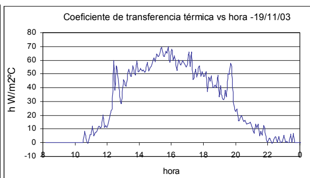
Figura 4. h vs hora para el día 19/11/03.
