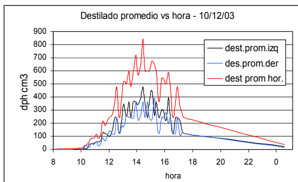
Figura 6. Volumen destilado por el vidrio izquierdo, derecho y total, el 10/12/03.
