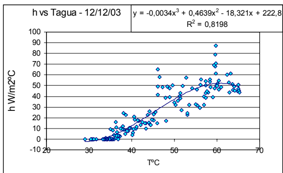
Figura 3. h vs Tagua y ajuste para el día 12/12/03.
