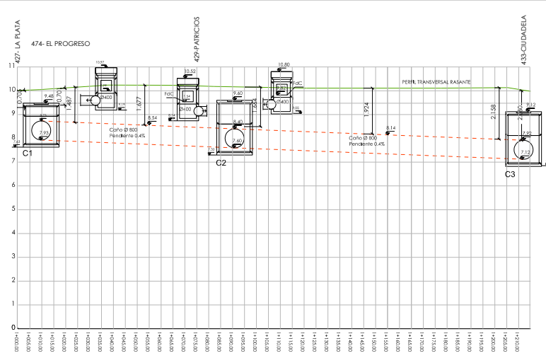
PERFIL LONGITUDINAL CALLE EL PROGRESO ESC. HORIZONTAL 1:1000 ESC. VERTICAL 1:100
