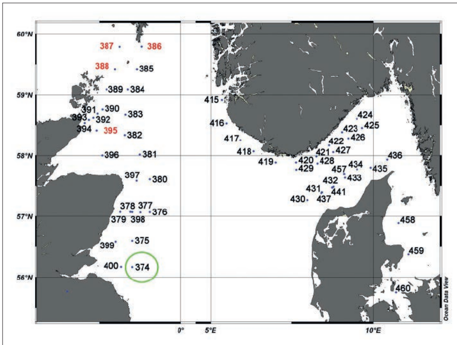
Abb. 3: Stationen der Nordsee Expedition 2007. Schwarze Stationsnummern zeigen AZA-1 im Plankton an, an Stationen mit roten Nummern wurde kein AZA-1 detektiert. Station 374 war die Station mit den höchsten AZA-1 Werten.
