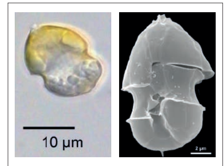
Abb. 4: Lichtmikroskop- (links) und Raster-elektronenmikroskopaufnahme (rechts) des AZA Produzenten Azadinium spinosum .
