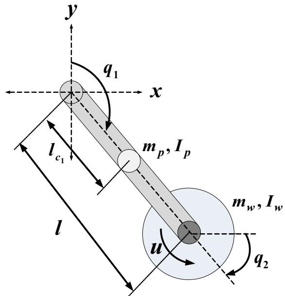
Fig. 1. The inertia wheel pendulum.
