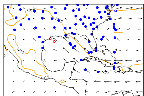
(d) CERA-20C
