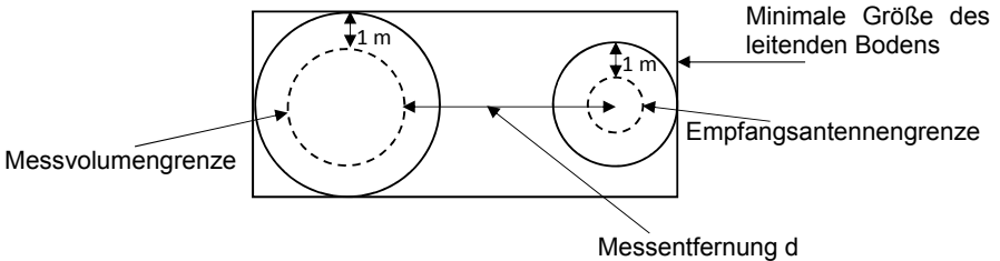
Bild 2.1: minimale Größe des leitenden Bodens
