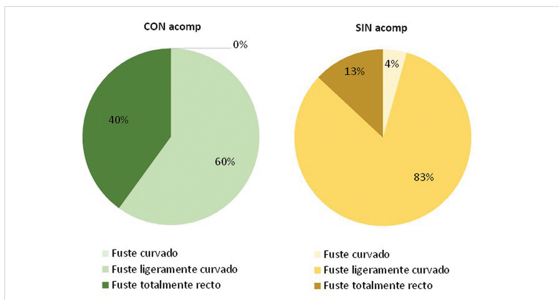
Figura 3. Porcentaje de nogales en relación a la rectitud del fuste CON y SIN acompañamiento de avellano en CALDES. Evaluación realizada a los 5 años de edad.
