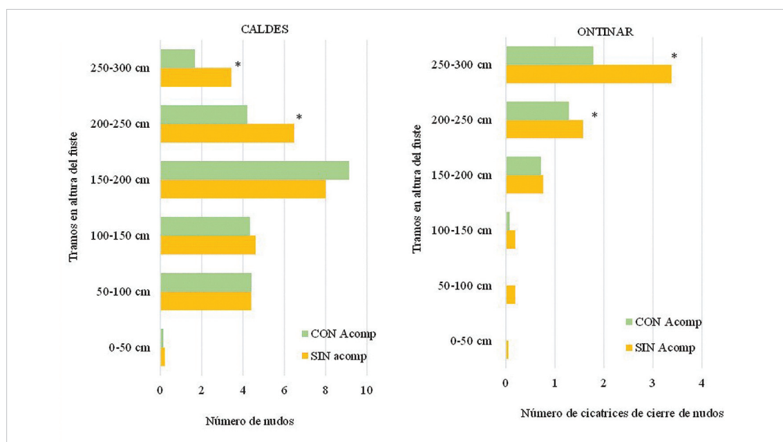
Figura 4. Número de nudos observados sobre el primer tramo de fuste de 3 m en CALDES hasta los 8 años (izquierda) y número de cicatrices procedentes del cierre de nudos en ONTINAR a los 10 años (derecha).
