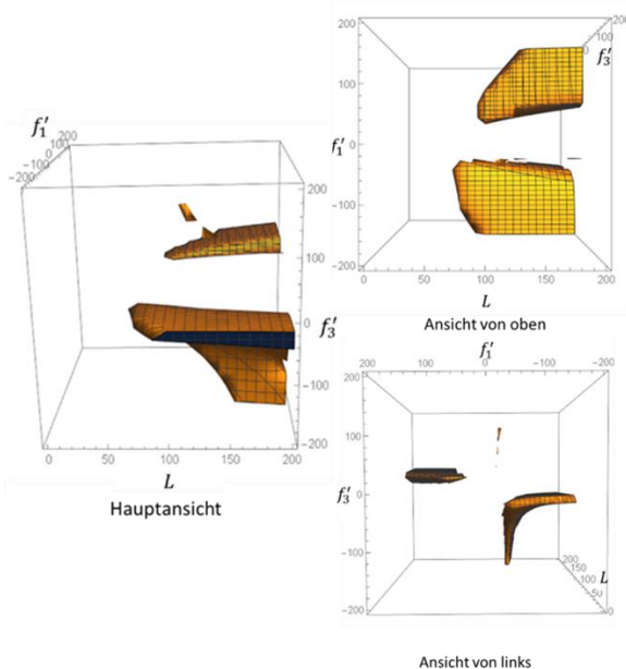
Abb. 3 Plot des Lösungsraums der betrachteten hybriden Zoomoptik in drei Ansichten
