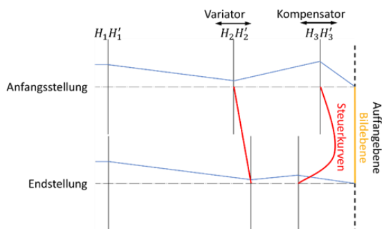
Abb. 1 Kollineares Startsystem einer klassischen Zoomoptik
