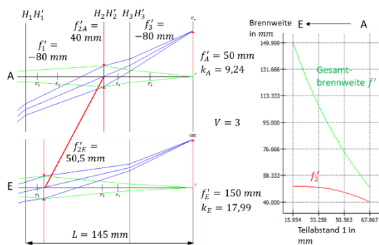
Abb. 4 Daten des gewählten hybriden Fotozoomobjektivs, dargestellt im Programm PARAX
