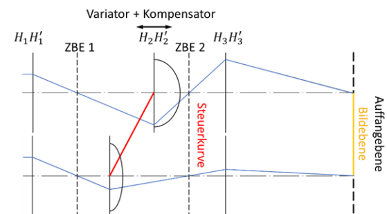
Abb. 2 Kollineares Startsystem eines möglichen hybriden Fotozoomobjektivs
