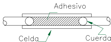
Fig. 5: Detalle de fijación de celdas solares
