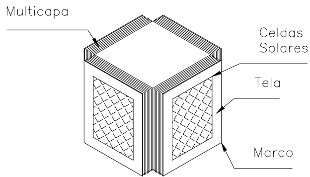
Fig. 6 Nano sat con multicapa
