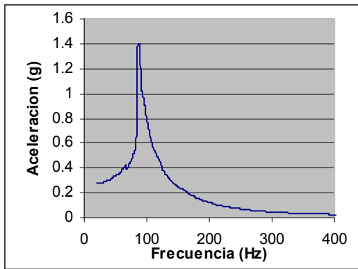
Fig.10: respuesta en frecuencia de panel encordado
