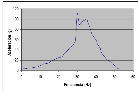
Fig.11 respuesta en frecuencia de panel entelado
