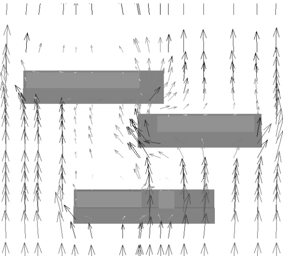
Figura 2: Planta con estudio de movimiento de aire en espacios exteriores y sobre fachadas con el fin de verificar las condiciones de ventilación cruzada.
