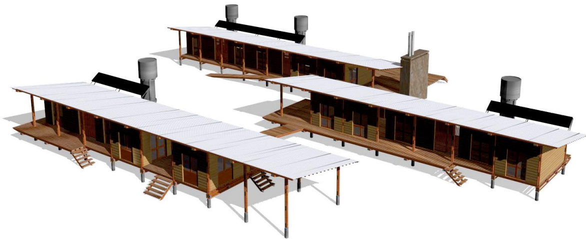
Figura 1: Vista del conjunto edilicio desde en Noroeste, elevado sobre el nivel del terreno, instalaciones solares correspondiente a la primera etapa de diseño, expansiones con mosquiteros y circulaciones cubiertas que permiten facil desplazamiento sin barreras, con gran importancia de los espacios intermedios.
