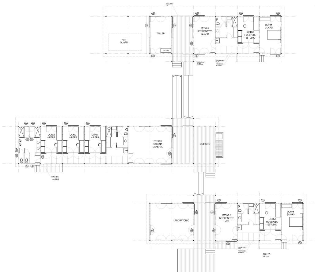
Figura 4: Planta del proyecto con los tres elementos unidos por una circulación techada en el sentido N - S: 1. Casa de Guardaparques, con garage y taller. 2. Casa de los Investigadores, con estar general y quincho en el sector central. 3. Casa del Director, con estudio o habitación de huéspedes y Laboratorio.
