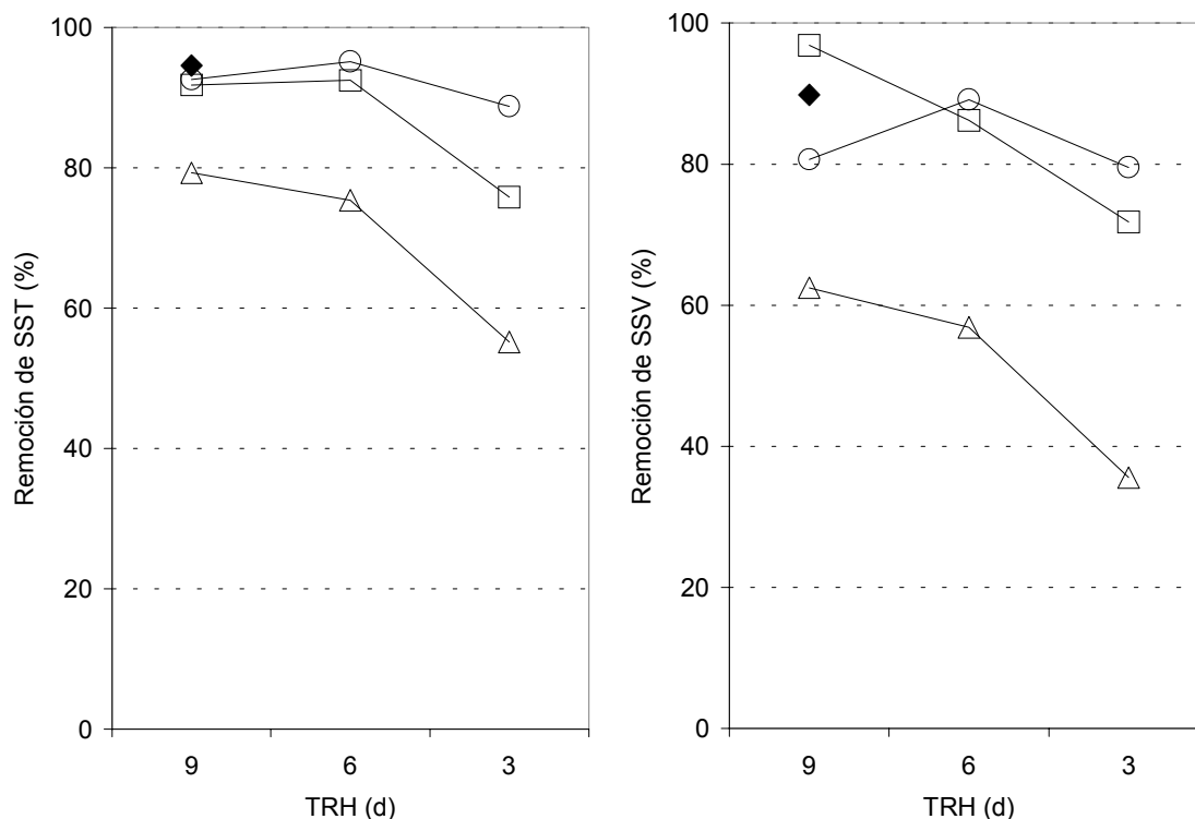
Figura 1. Remoción porcentual de SST y SSV a distintos TRH y para distintas alturas del manto de lodos: \blacklozenge = 1.84 m (100%); \square = 1.38 m (75%); \circ = 0.92 m (50%); \Delta = 0.46 m (25%).
