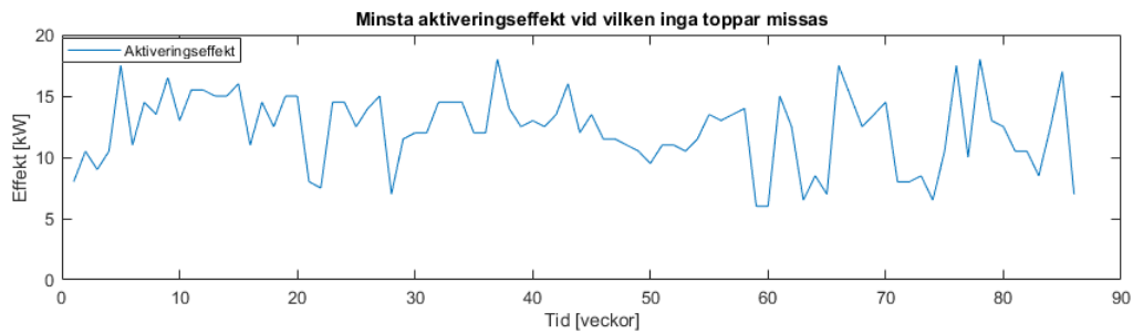
Figur 4: Variation av simulerade saltvattenbatteriets aktiveringseffekt över tid på Jarlaparkens förskola
