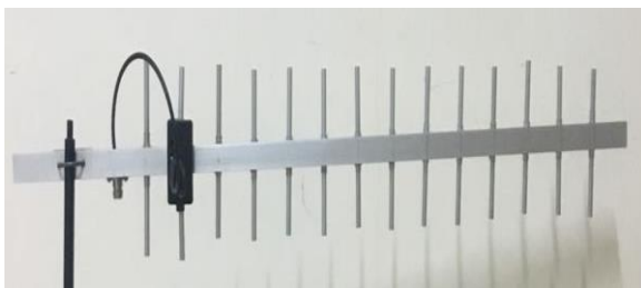
Gambar. 4 Antena yagi 14 Elemen
