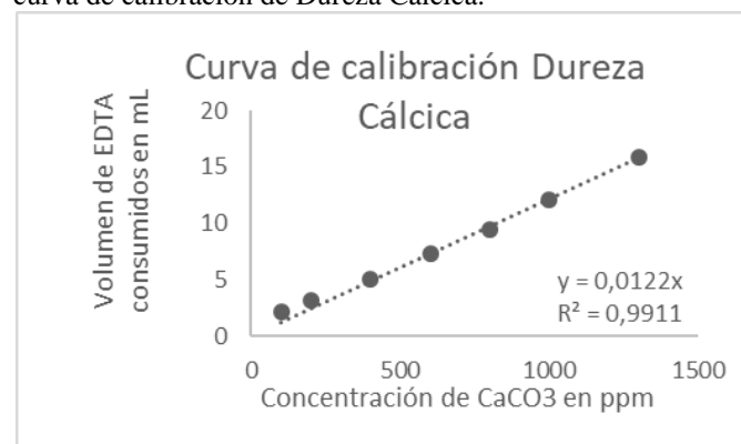
Gráfica 2. Curva de calibración correspondiente a Dureza Cálctica
