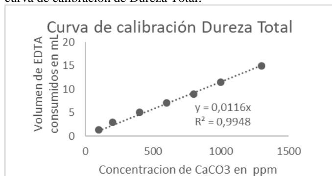
Gráfica 1. Curva de calibración correspondiente a Dureza Total
