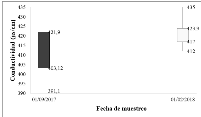
Gráfica 4. Variación en la Conductividad eléctrica
