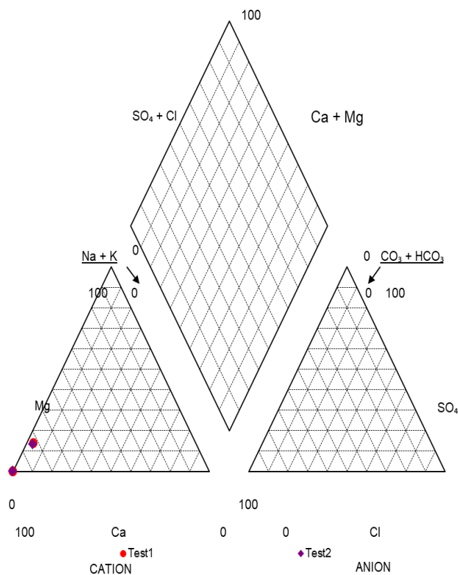
Figura 4. Representación Iónica del agua mineral La Calera en el Diagrama Hidroquímico de Piper.
