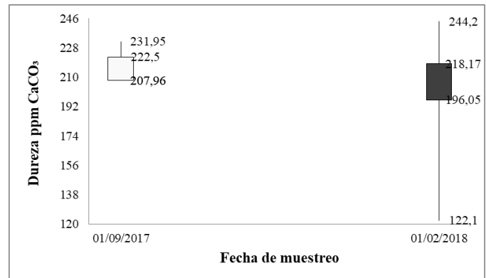
Gráfica 7. Variación de la Dureza
