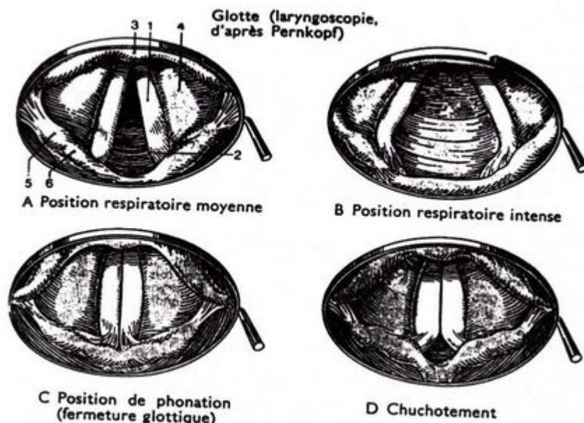
FIGURE 1.2 – Coupe latérale du larynx, montrant quatre positions différentes des cordes vocales : a) glotte ouverte ; b) glotte largement ouverte ; c) glotte fermée, d) glotte entrouverte, (Pernkopf, 1952)
